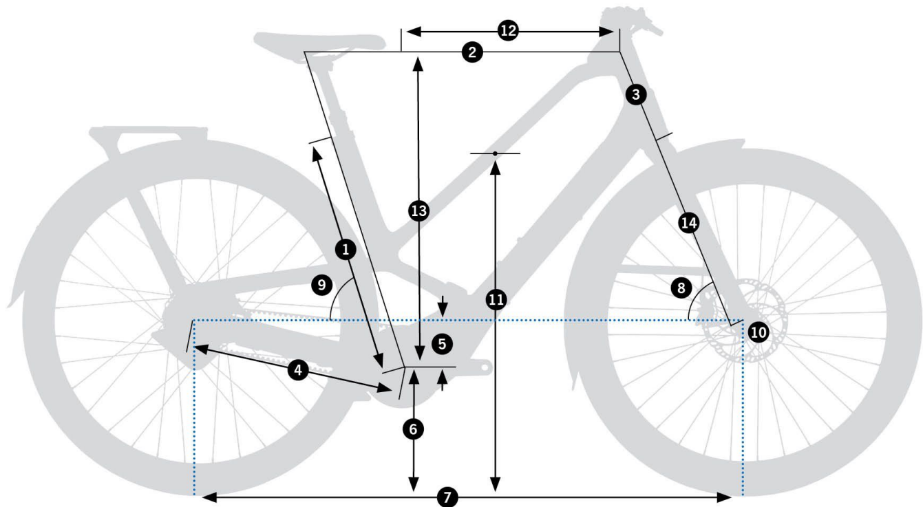
Schemat pomiarowy geometrii Orbea Diem 20
