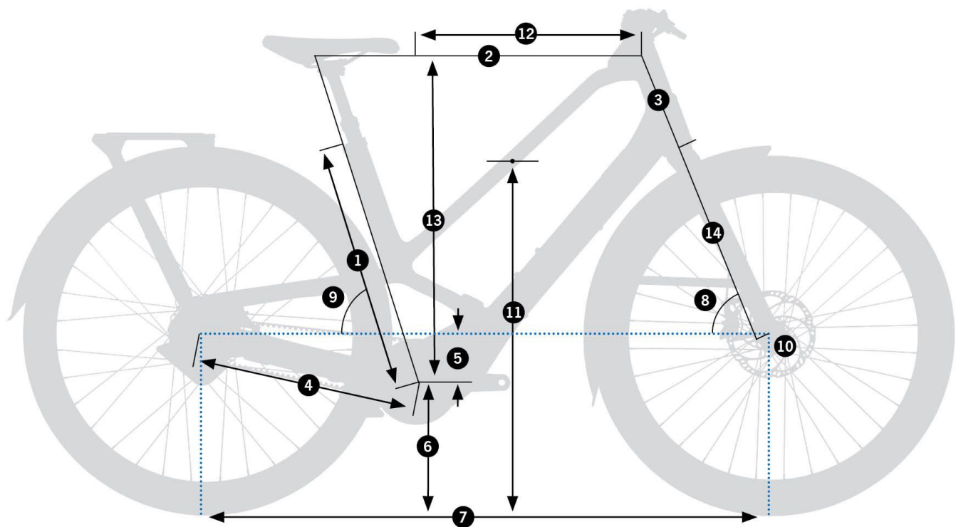
Schemat pomiarowy geometrii Orbea Diem 10
