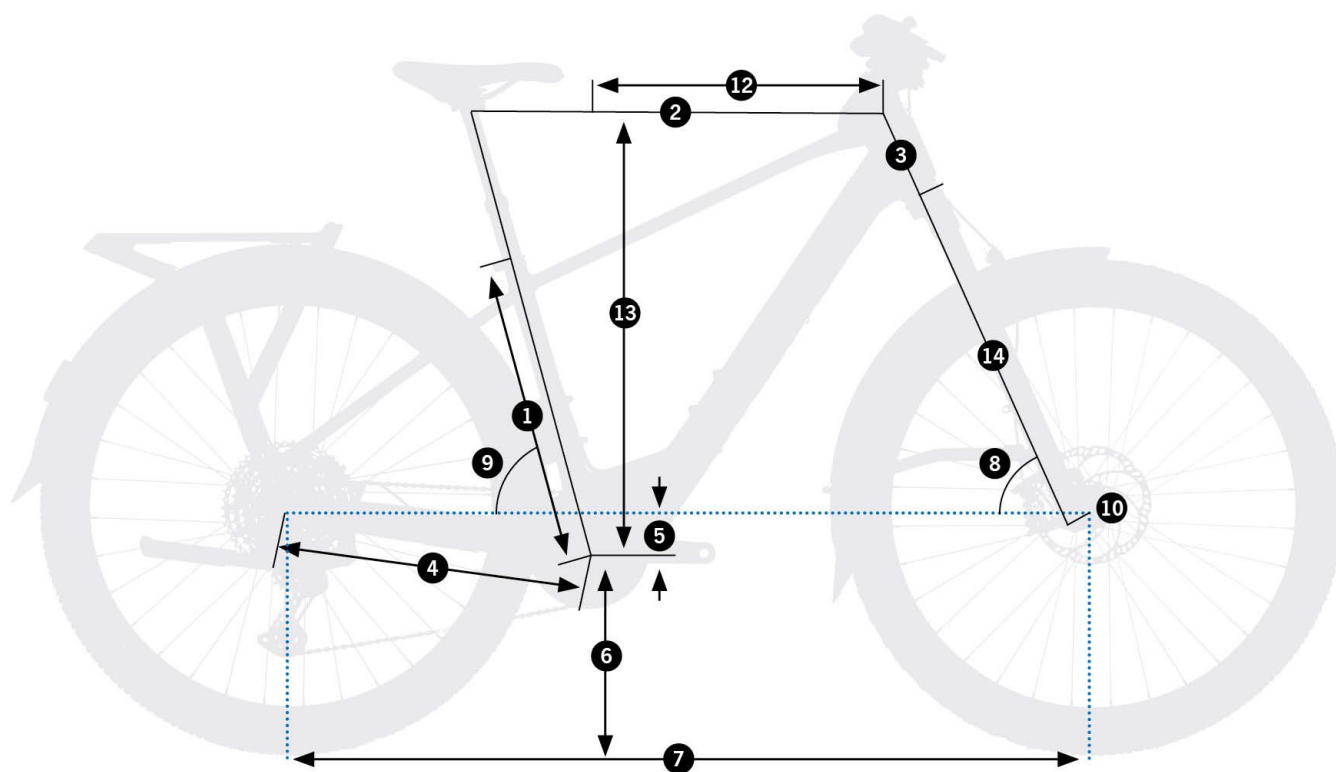
Schemat pomiarowy geometrii Orbea Kemen ADV 10
