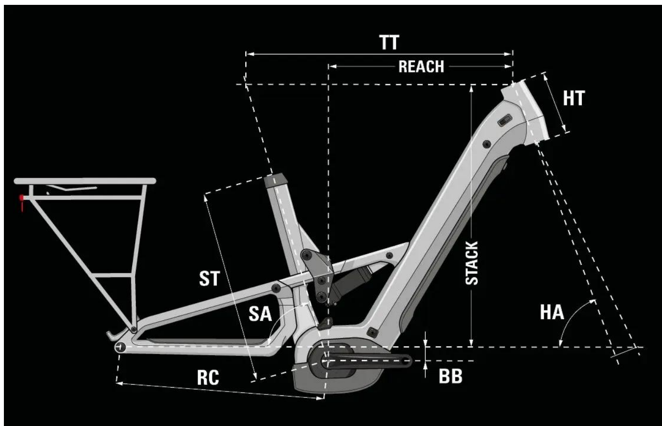
Schemat pomiarowy geometrii Lapierre E-Explorer FS (Low)
