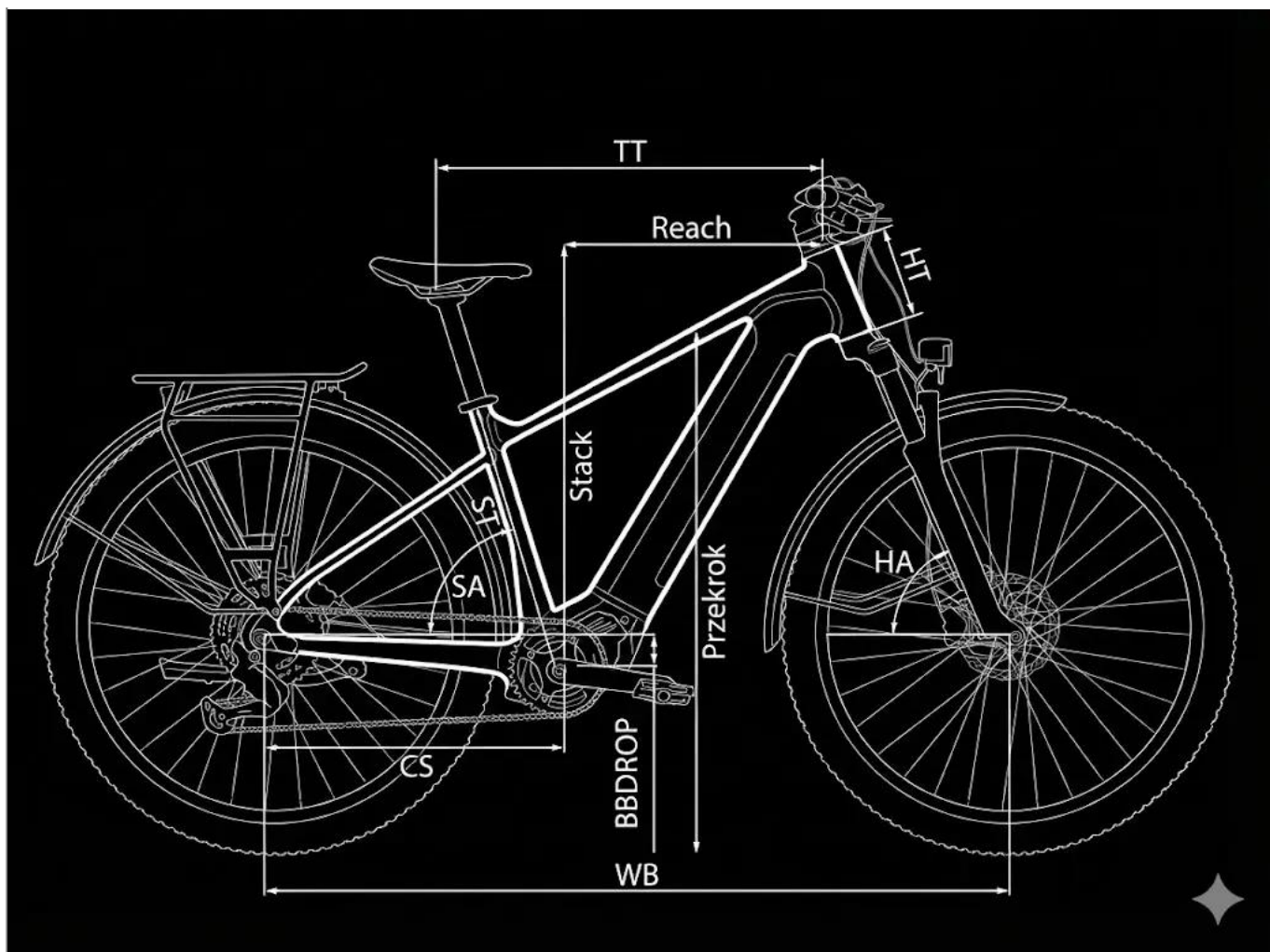
Rysunek techniczny - geometria ramy Influx SUV Hybrid
