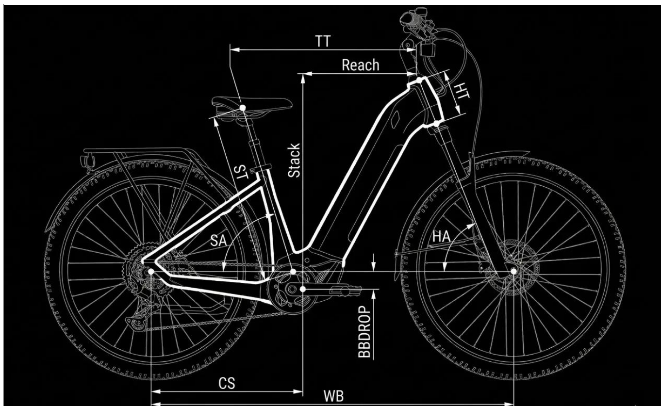
Rysunek techniczny - wymiary ramy Estima COMP
