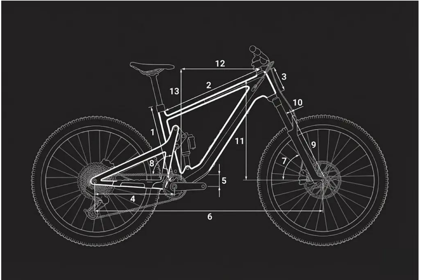
Schemat pomiarowy geometrii Ghost Path Riot CF
