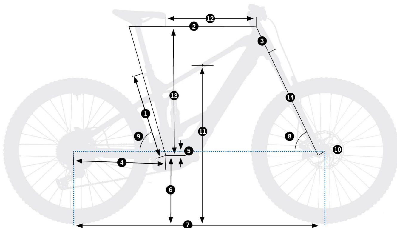
Wild H20 – schemat geometrii ramy (źródło: Orbea)
