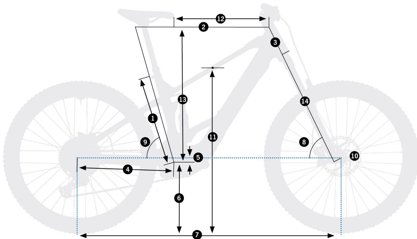
Wild ST H30 – schemat geometrii ramy (źródło: Orbea)
