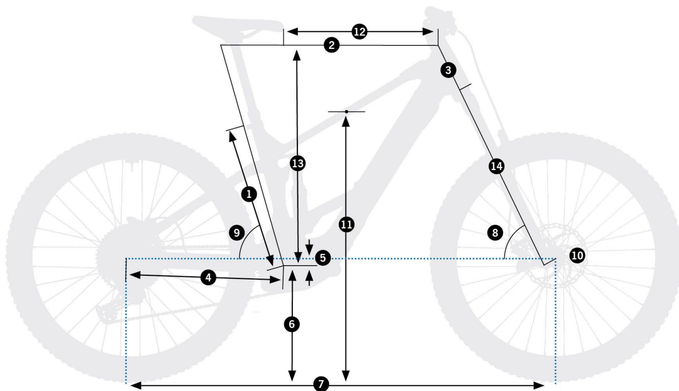
Schemat pomiarowy geometrii Orbea Wild ST
