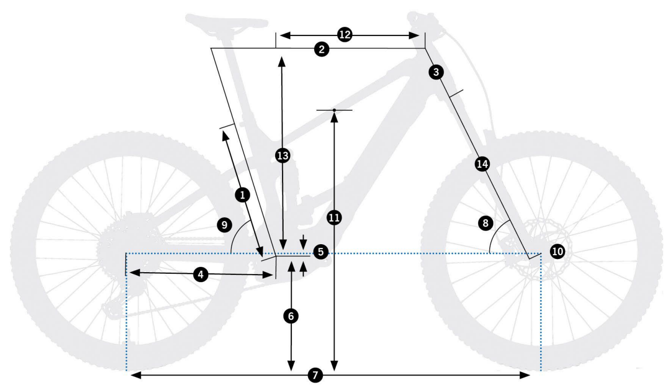
Wild M20 – schemat geometrii ramy (źródło: Orbea)
