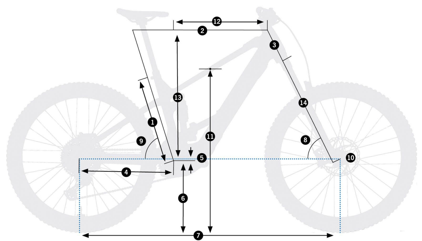
Wild M-LTD – schemat geometrii ramy (źródło: Orbea)
