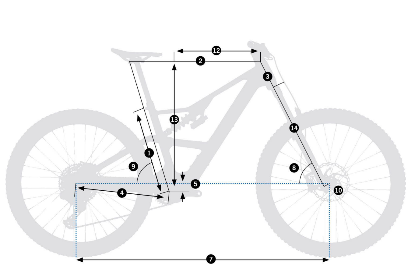
Rise LT M20 2026 – schemat geometrii ramy (źródło: Orbea)
