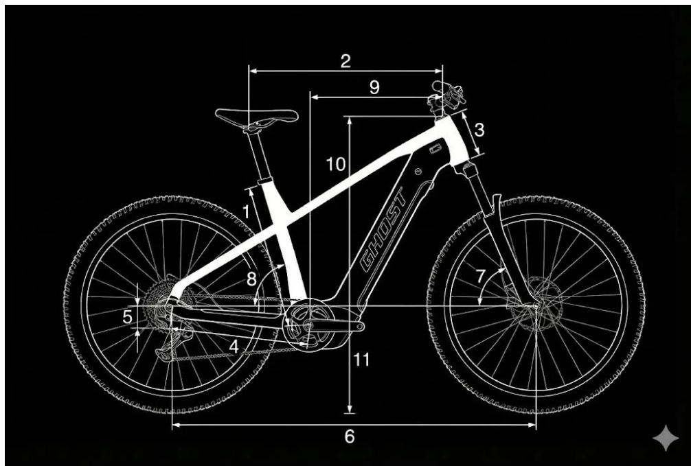
Rysunek techniczny – geometria Ghost E-Teru
