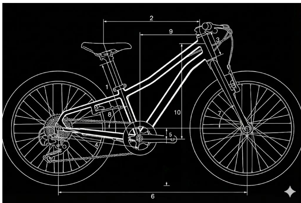
Rysunek techniczny – geometria ramy (20" Pro)
