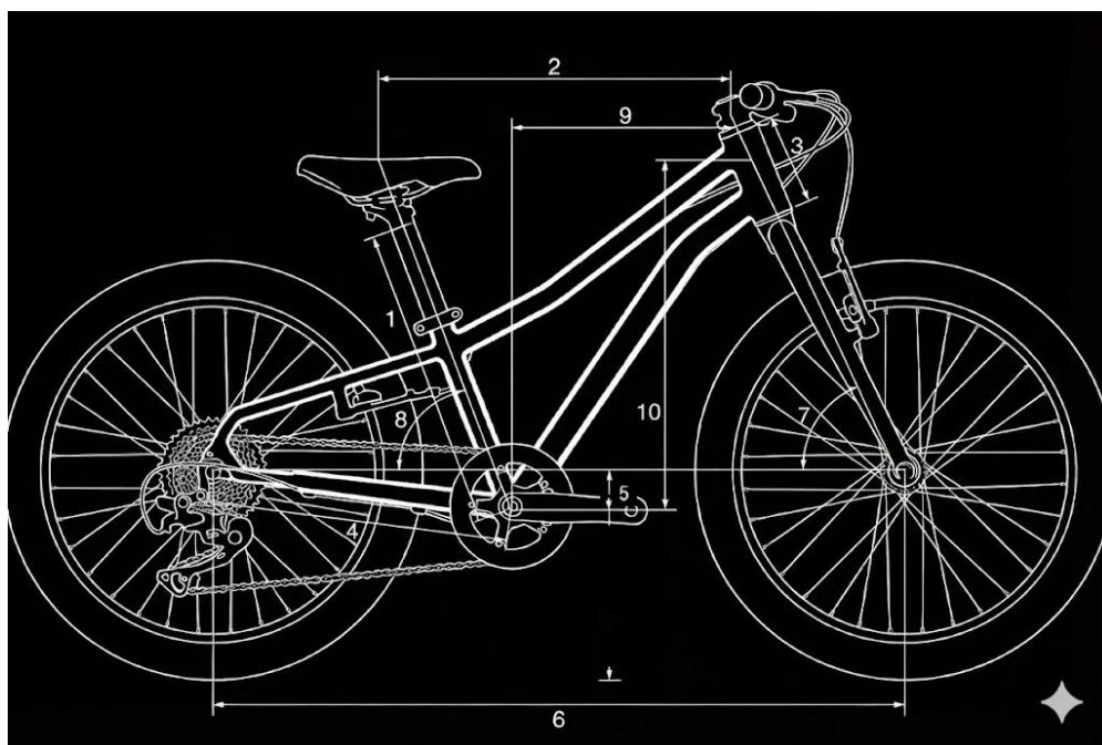
Rysunek techniczny – geometria ramy (20" Pro)
