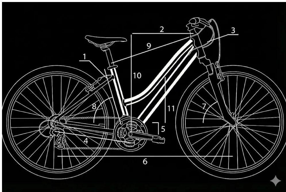
Rysunek techniczny – geometria ramy damskiej
