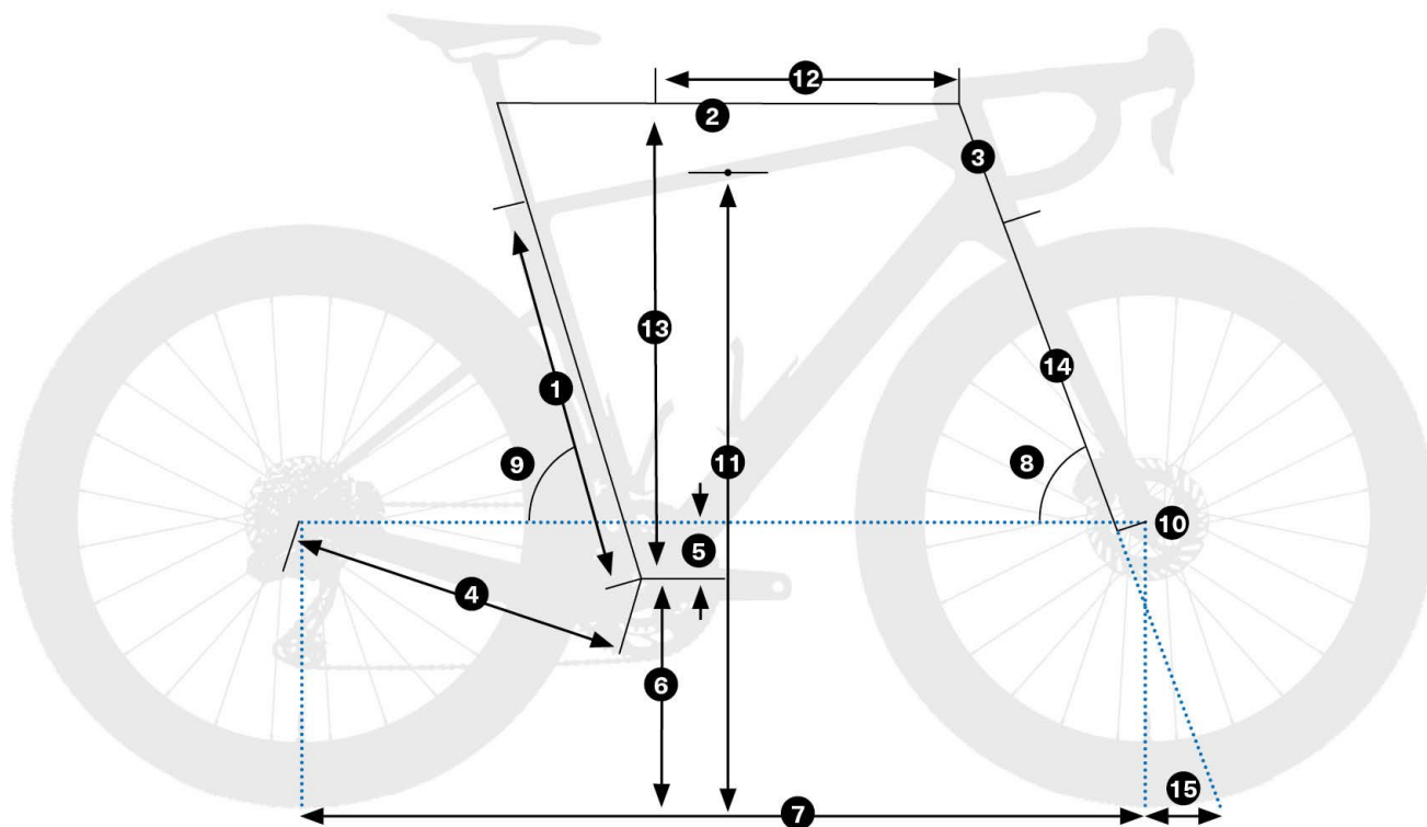
Schemat pomiarowy geometrii Orbea Terra Race M21eLTD 1X 2026
